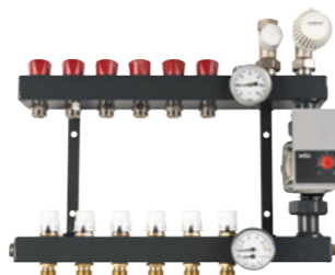
Boxer-CF (art.nr. bovenaansluiting: 50.402 t/m 50.415 en art.nr. onderaansluiting: 50.452 t/m 50.465)
