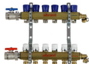
Messing-CF (art.nr. 54.202 t/m 54.215) 2 t/m 15 groepen leverbaar
