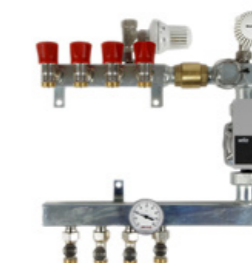
LCV+-S (art.nr. 52.922 t/m 52.930)
