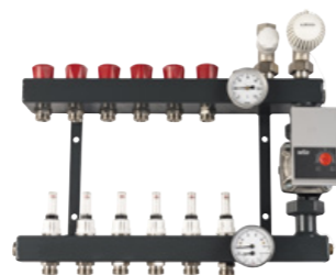
Boxer-FL (art.nr. bovenaansluiting: 50.202 t/m 50.215 en art.nr. onderaansluiting: 50.252 t/m 50.265)
