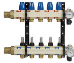
2010 MA (art.nr. 55.202 t/m 55.212) 2 t/m 12 groepen leverbaar
